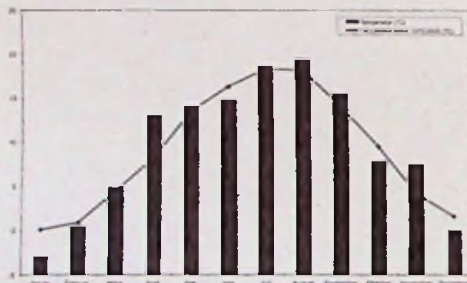
Abb. 4: Monatliche Niederschläge im Jahr 2009 in Dresden-Klotzsche.
