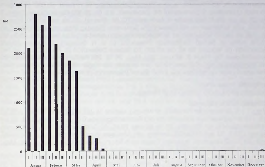
Abb. 15: Das Auftreten des Seidenschwanzes 2006 in Sachsen nach Summe der Dekadenmaxima je Gebiet.
